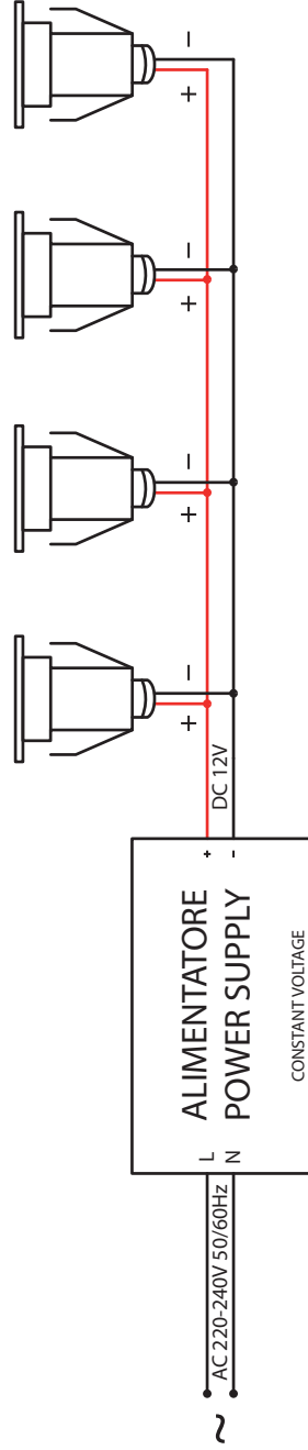
SCHEMA DI COLLEGAMENTO/CONNECTION DIAGRAM
